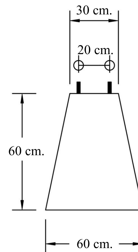
รูปขยายตอม่อ
