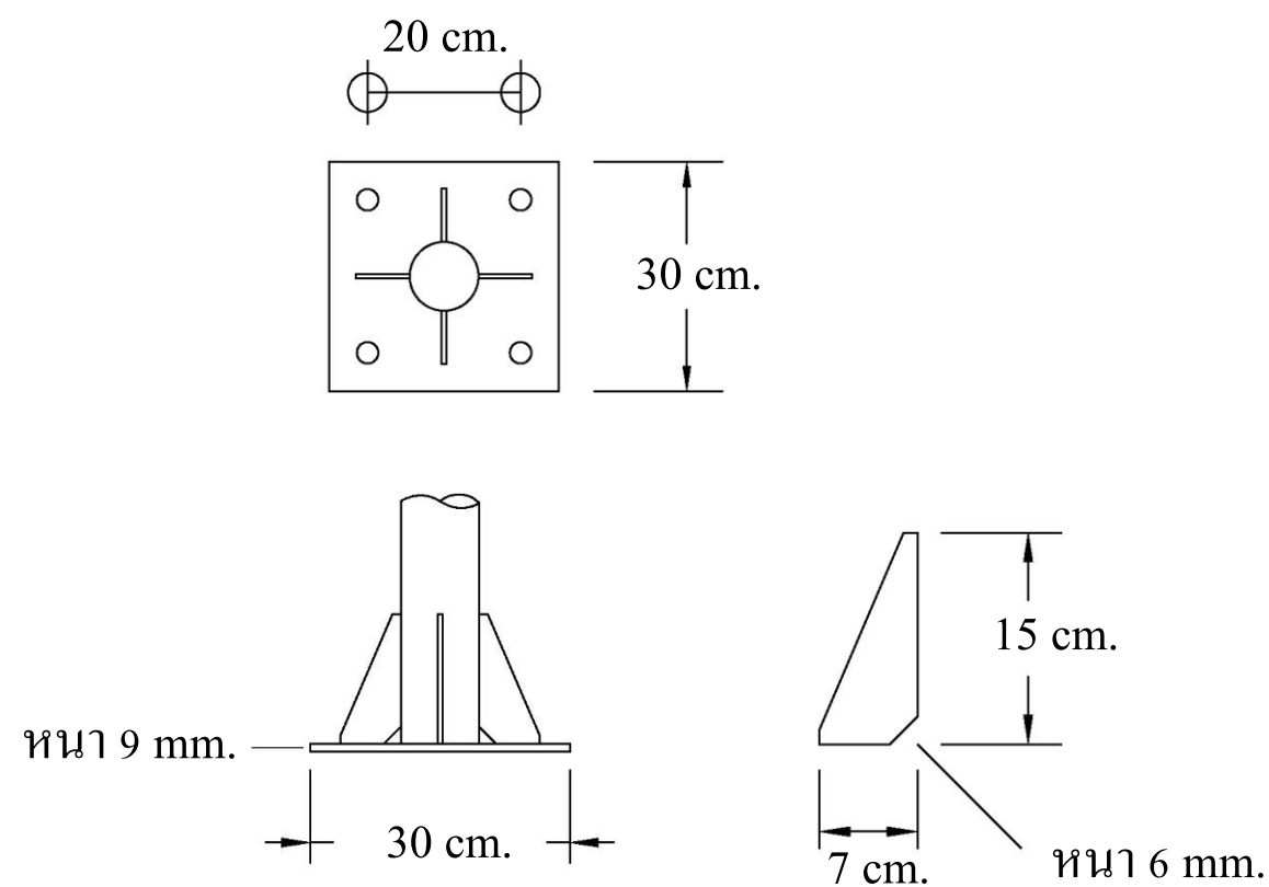
รูปขยายแผ่นเหล็กฐานเสา (Plate) และค้ำ
