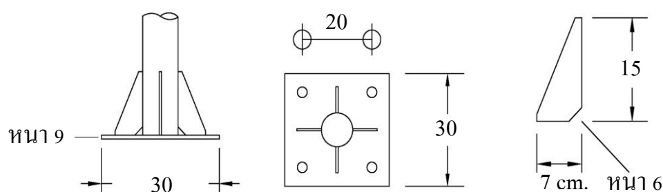
รูปขยายแผ่นเหล็กฐานเสา (Plate) และคิรบ
